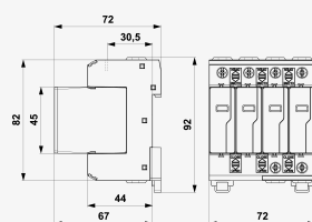
Rozměry
